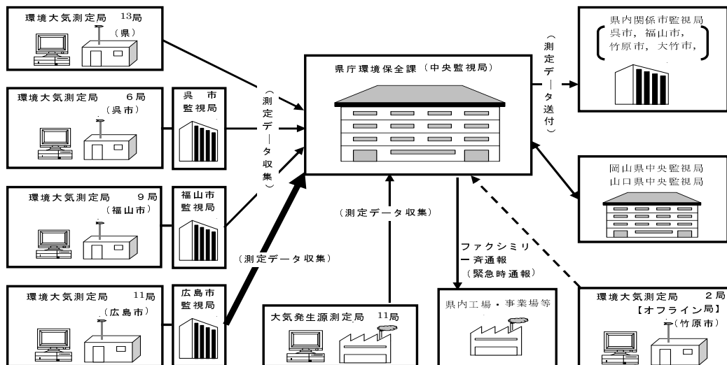
大気汚染常時監視システム系統図
