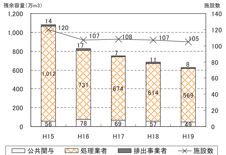
図表 2-1-7 産業廃棄物最終処分場の施設数及び残余容量
