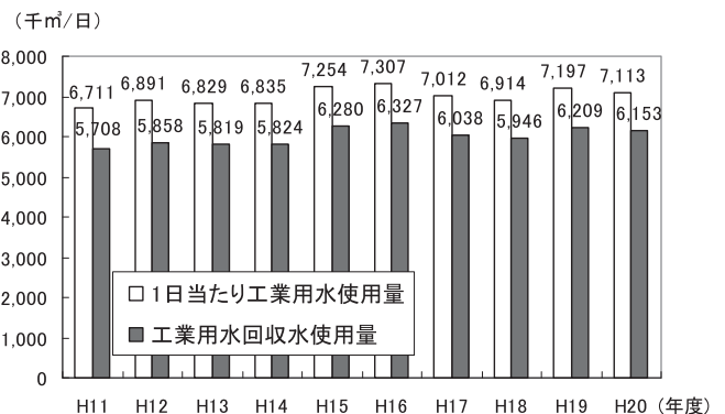
図表 2-1-15 1日当たり工業用水及び回収水使用量
