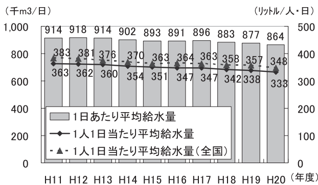
図表 2-1-14 1日及び1日1人当たり平均給水量（上水道事業のみ）
