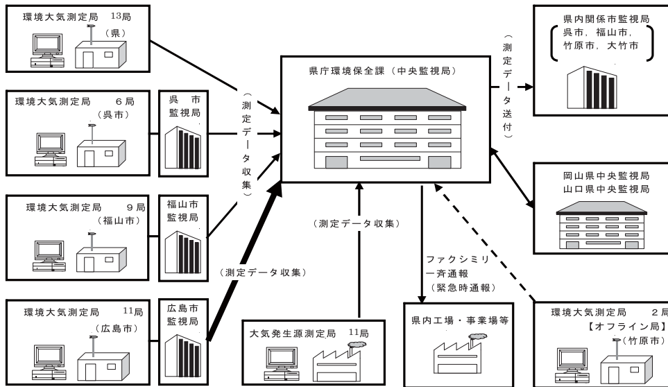
図表 2-2-6 大気汚染常時監視システム系統図
