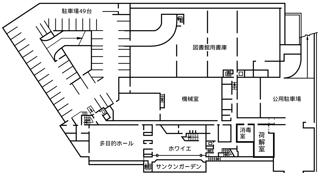
地下2階平面図
