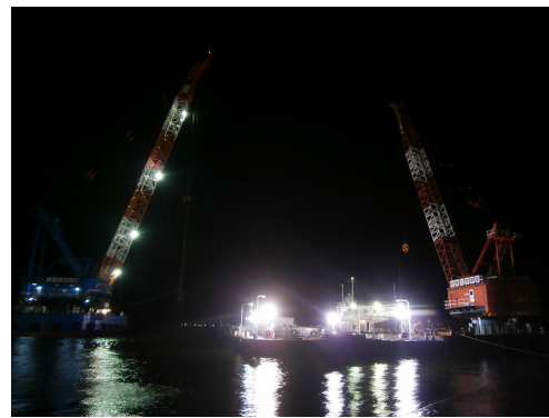
浮函を160t吊起重機船により移動させた後550t吊起重機船と交代
