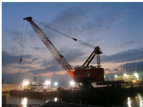
再び160t吊起重機船により、浮函を移設先に移動させ、チェーン碇係
