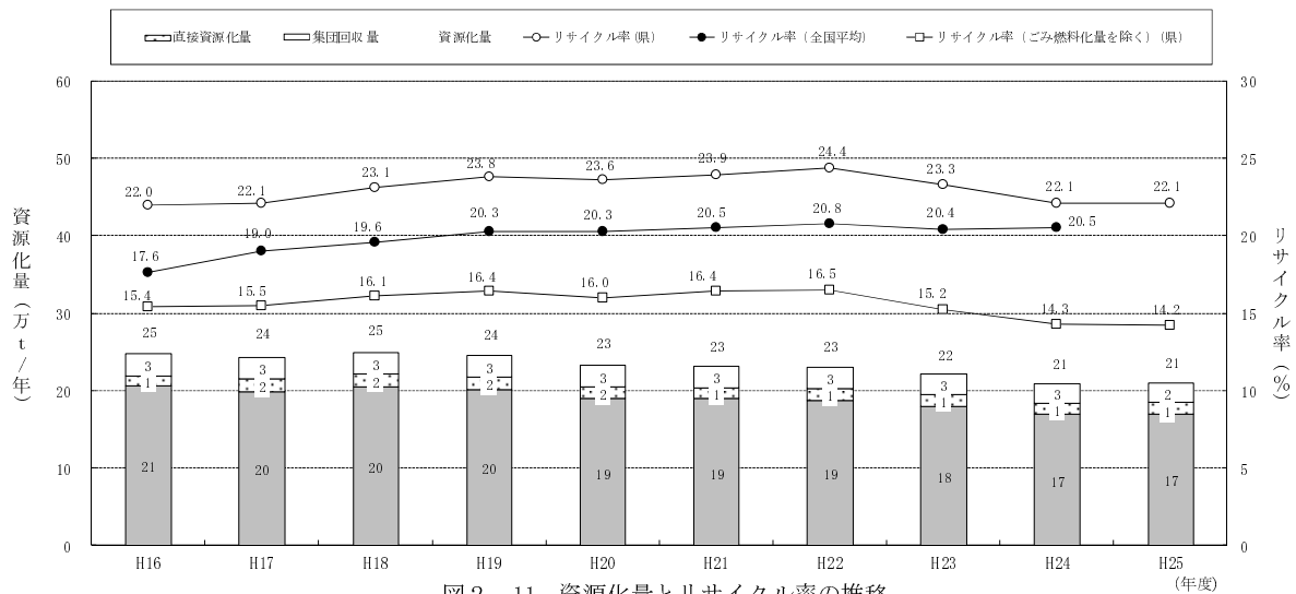
図 2-11 資源化量とリサイクル率の推移
