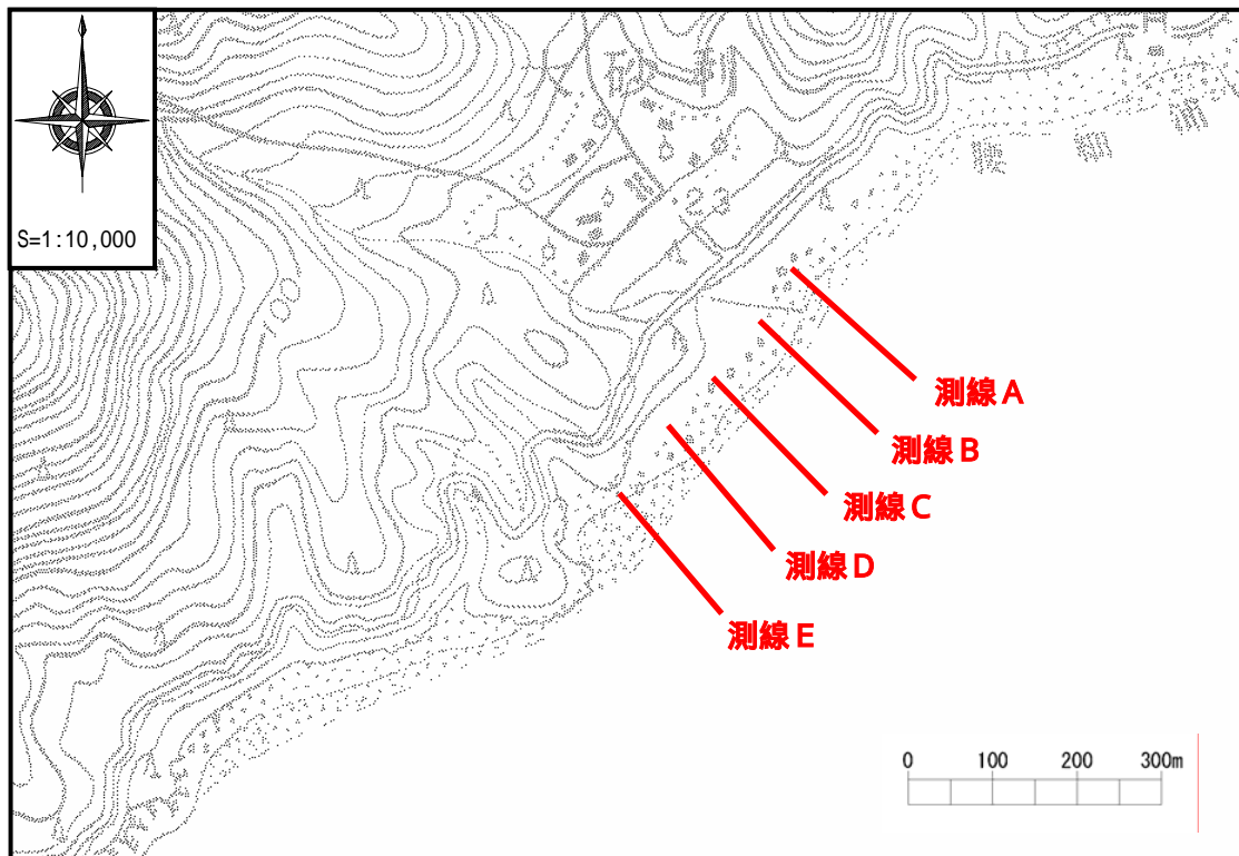
図4 調査測線位置図
