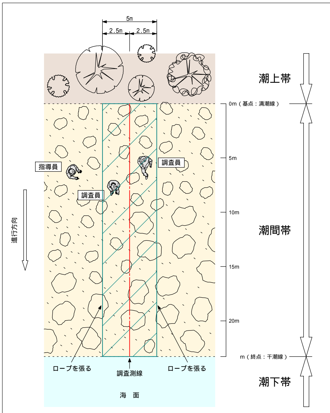
図5 調査方法模式図(平面図)
