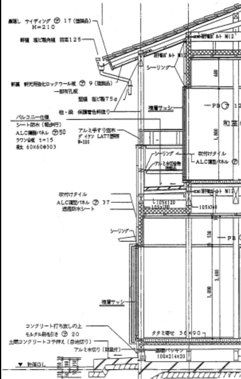
【建築物断面図】
