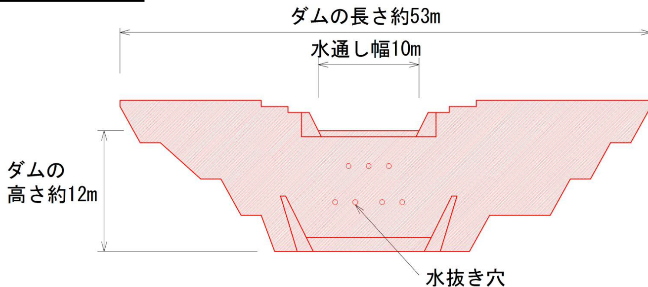
正面図
