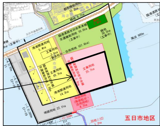
【広島港五日市地区 港湾計画図(H31.3改訂)】
