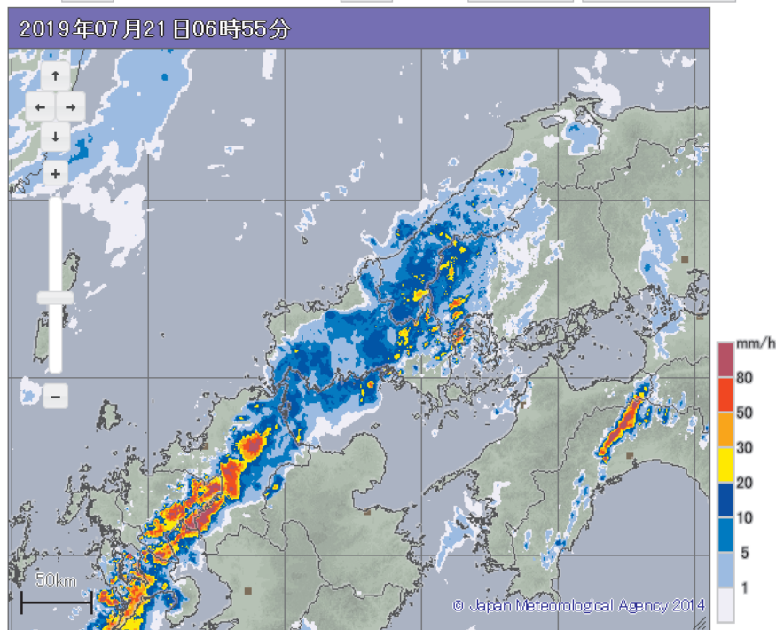
レーダー画像 (21日06時55分)
