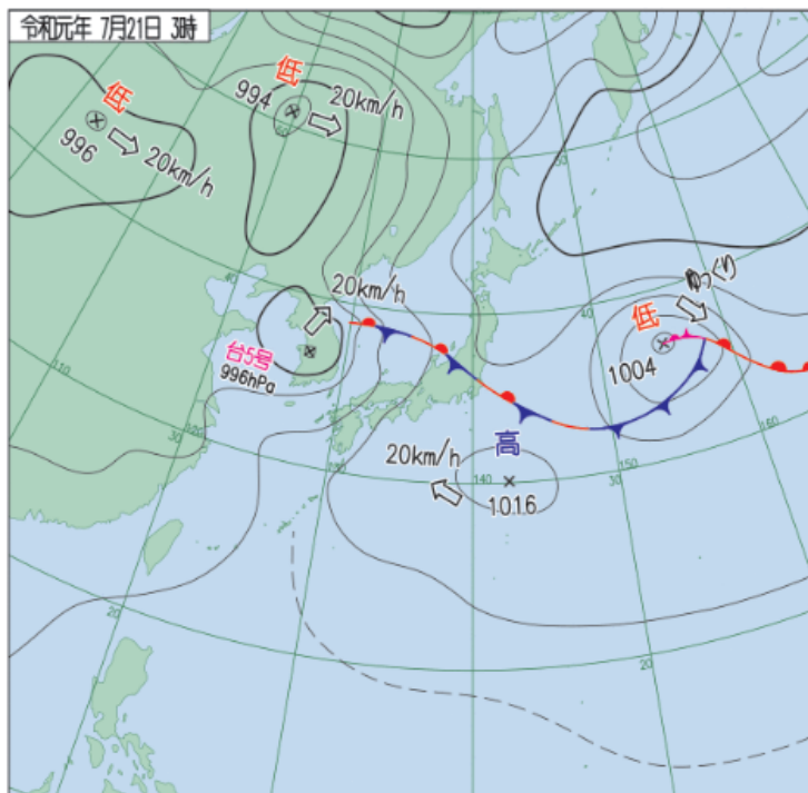
21日03時 地上天気図
