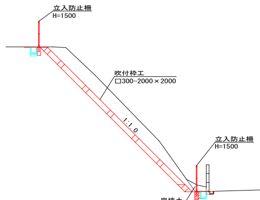
標準断面図
