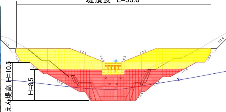
堰堤一般図
