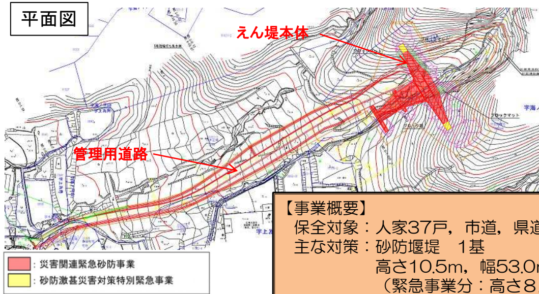
堰堤一般図
