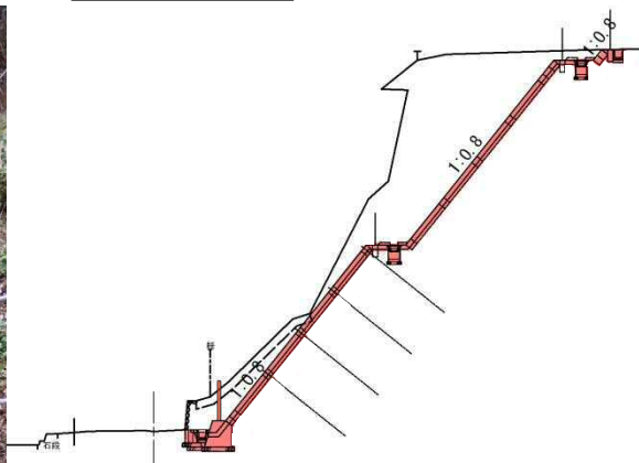
標準断面図
