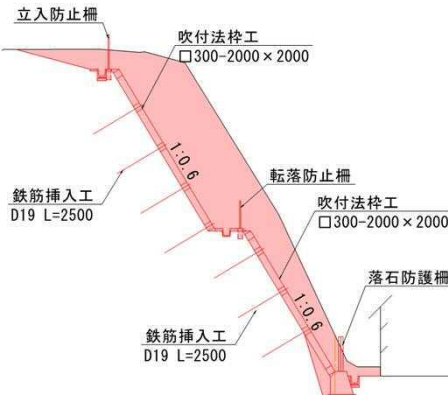
標準断面図
