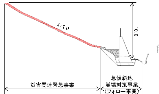
標準断面図
