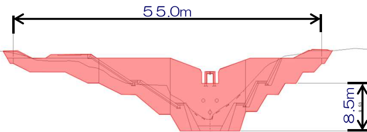
堰堤一般図
