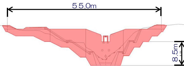
堰堤一般図
