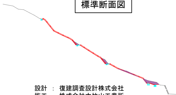
標準断面図
