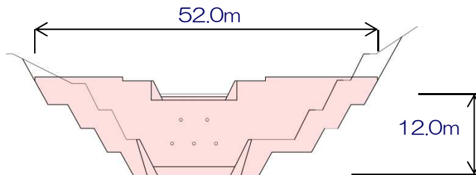
堰堤一般図
