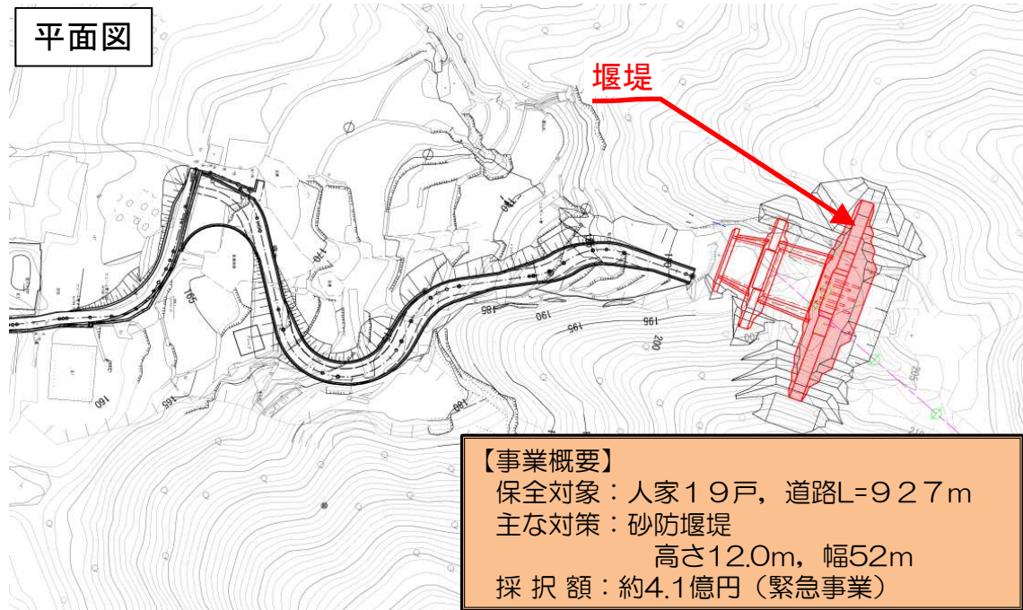
堰堤一般図
