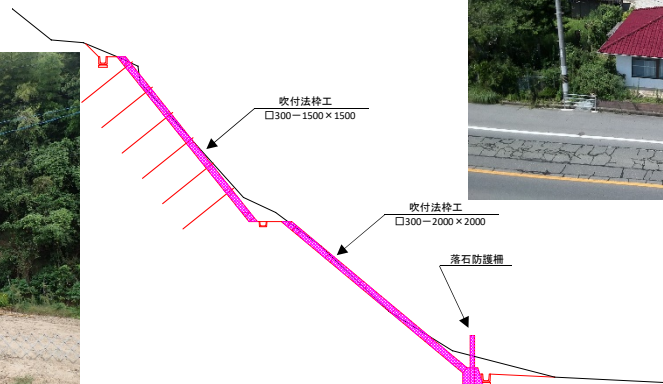
標準断面図
