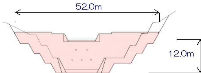
堰堤一般図
