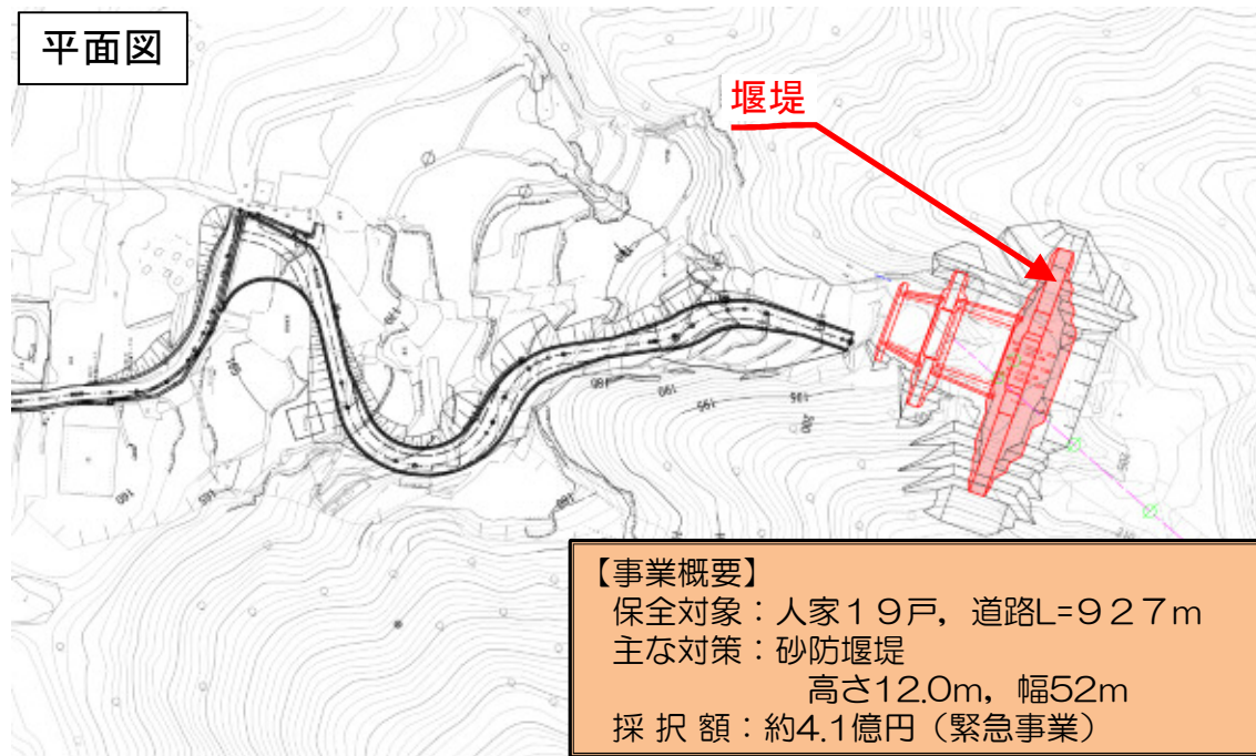
堰堤一般図
