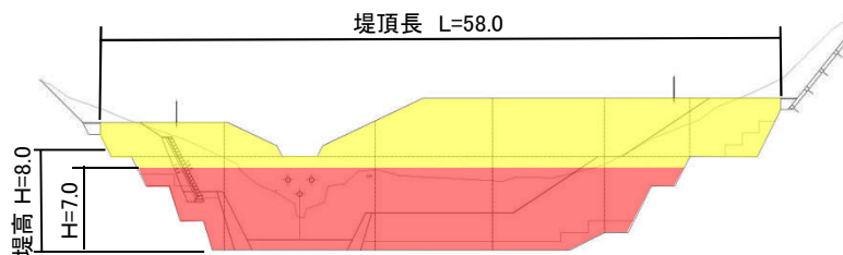
堰堤一般図
