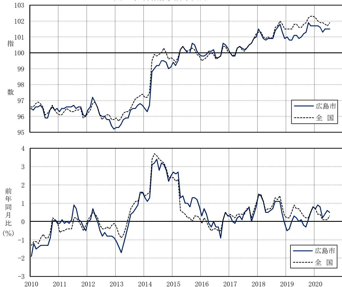
図1 総合指数, 前年同月比 2010.1~2020.7
