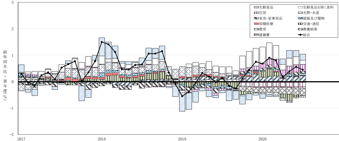
図5 総合指数の前年同月比に対する10大費目別寄与度の推移 2017.1～2020.7
