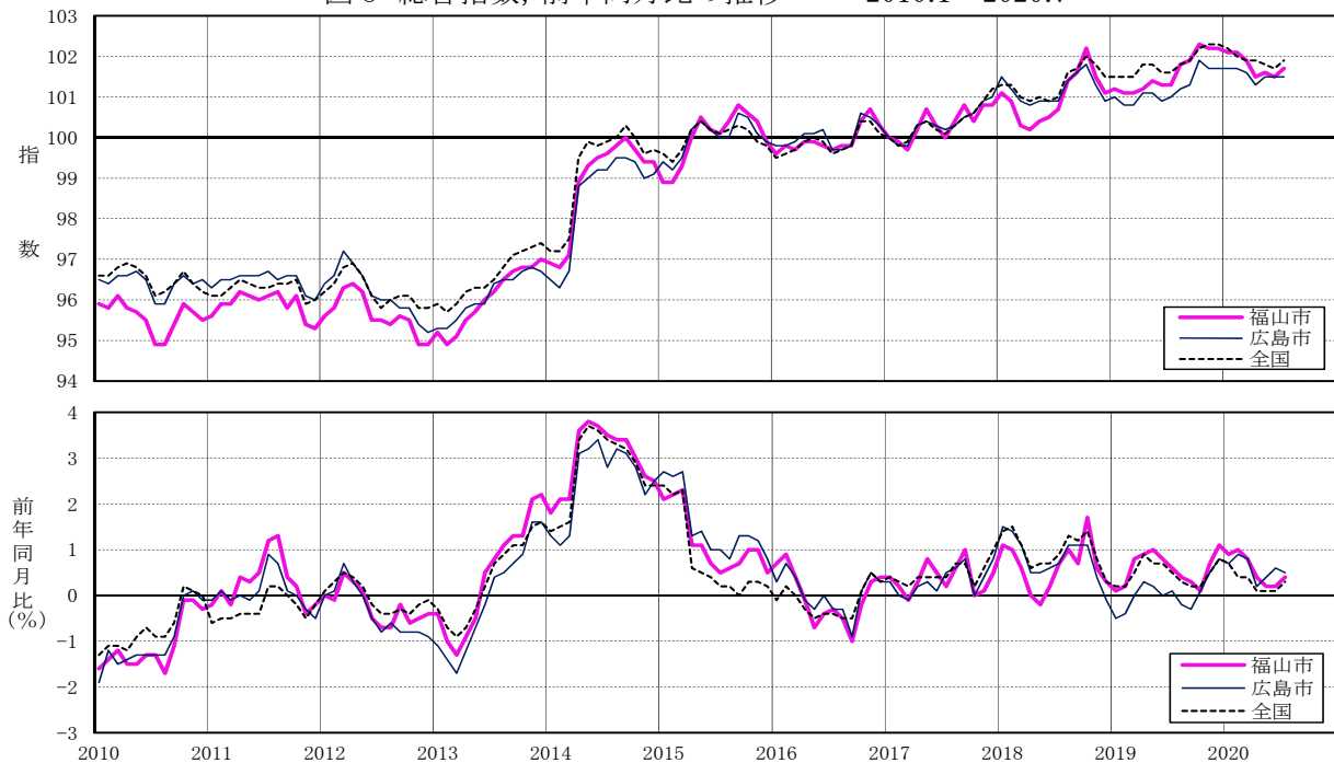
図8 総合指数, 前年同月比の推移 2010.1～2020.7
