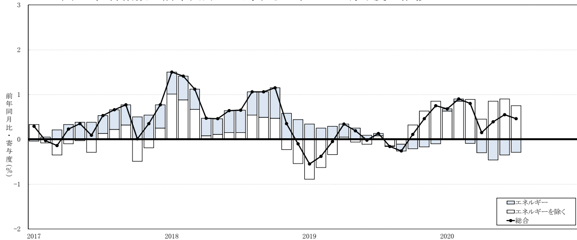
図6 総合指数の前年同月比に対するエネルギー寄与度の推移 2017.1～2020.7
