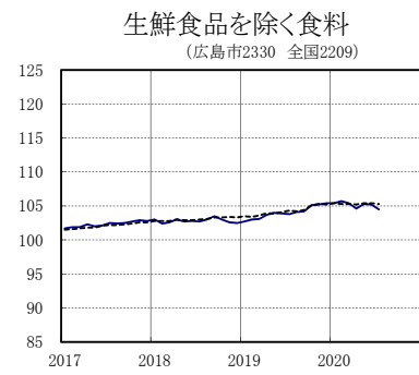
図7 10大費目指数の推移 2015年=100, 2017.1~2020.7
