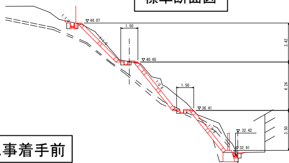
標準断面図
