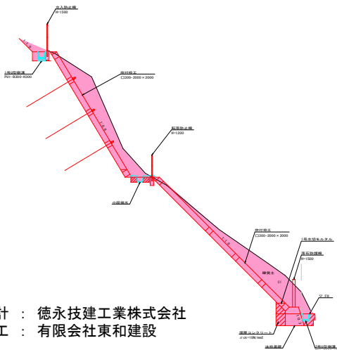
標準断面図
