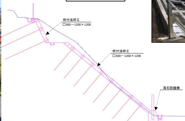
標準断面図
