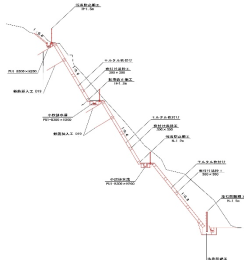
標準断面図
