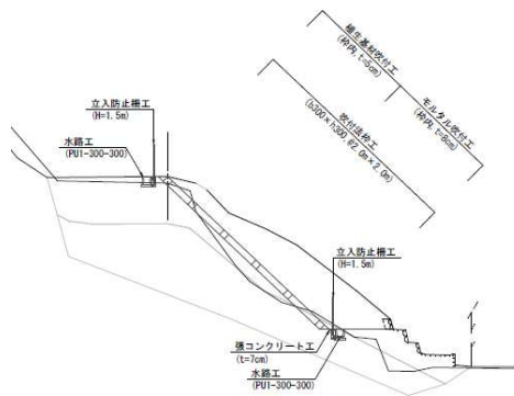
標準断面図
