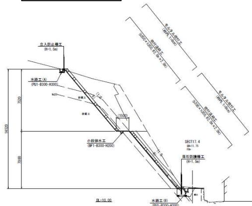
標準断面図
