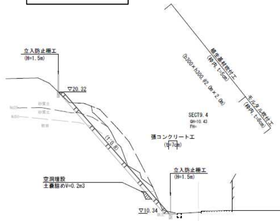
標準断面図
