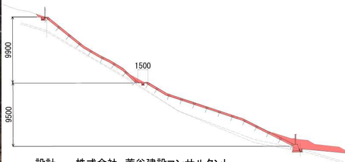
標準断面図
