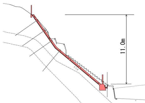
標準断面図
