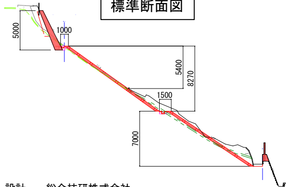
標準断面図
