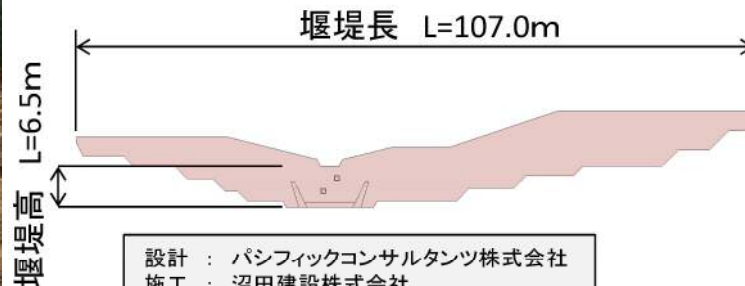
堰堤一般図
