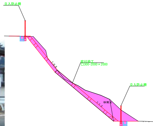
標準断面図
