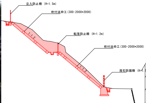
標準断面図
