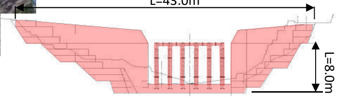
堰堤一般図
