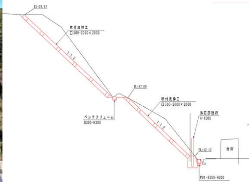
標準断面図
