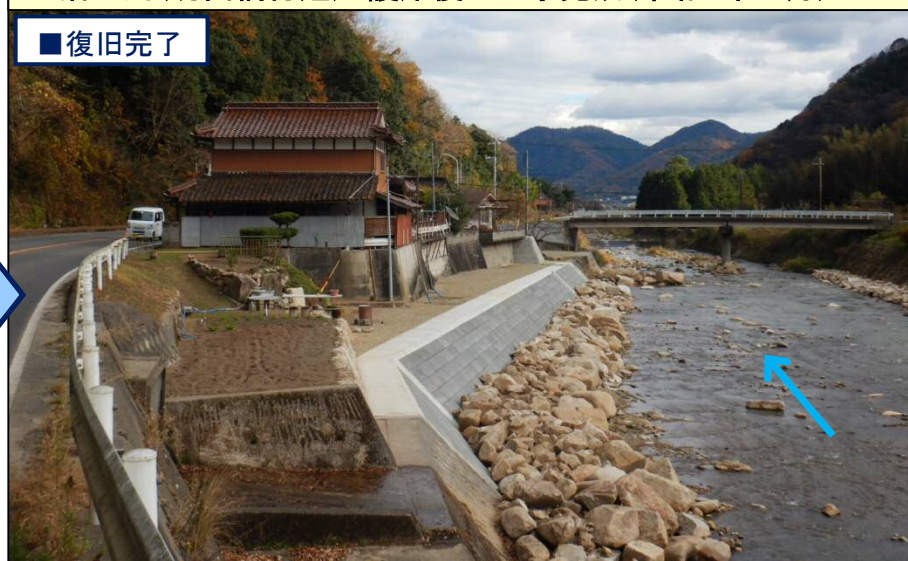
沼田川(切畠橋付近) 護岸復旧工事完成(令和2年11月)
