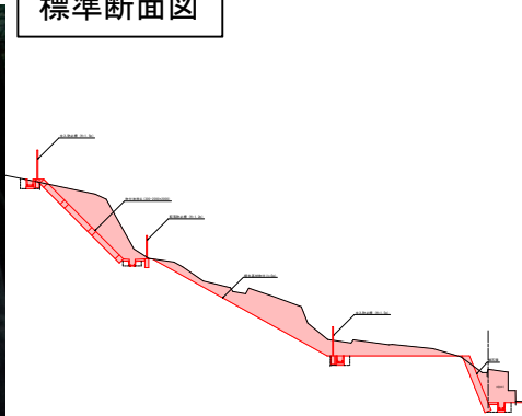
標準断面図
