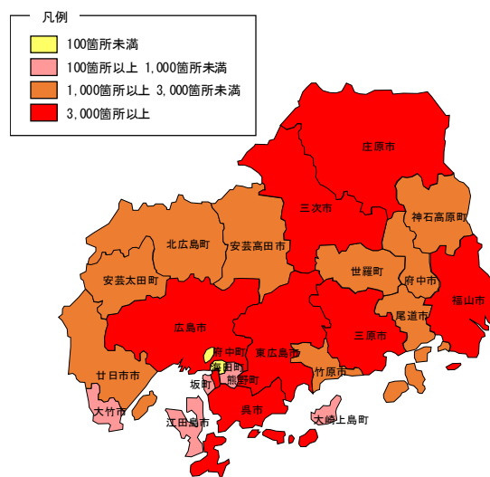
図 3-12 土砂災害警戒区域の指定状況
