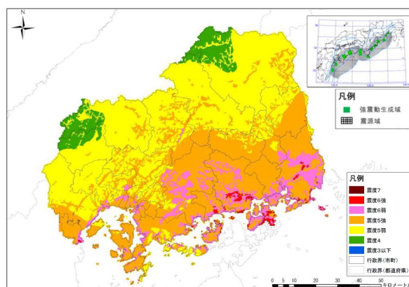
図 3-11 南海トラフ巨大地震(陸側ケース)の震度分布
