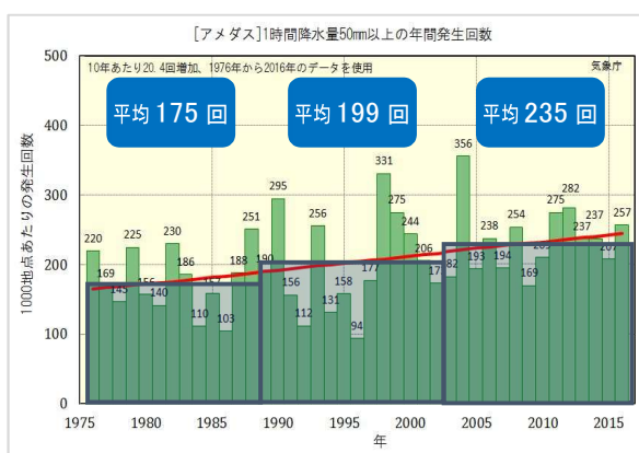
図 3-10 1時間降水量50mm以上の年間発生回数(全国)
