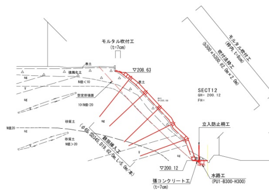
標準断面図
