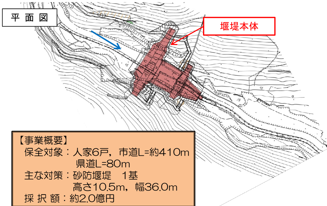
堰堤一般図
