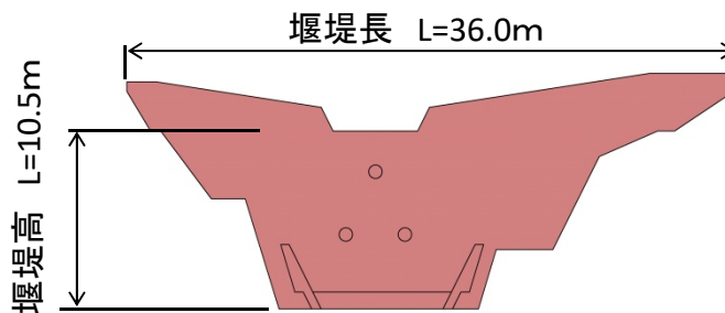
堰堤一般図
