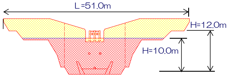
堰堤一般図
