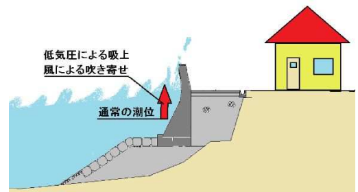
高潮対策事業のイメージ
