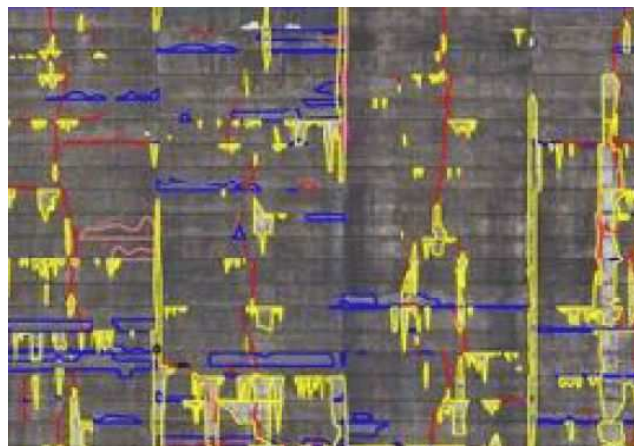
デジタル解析によるコンクリート損傷図
