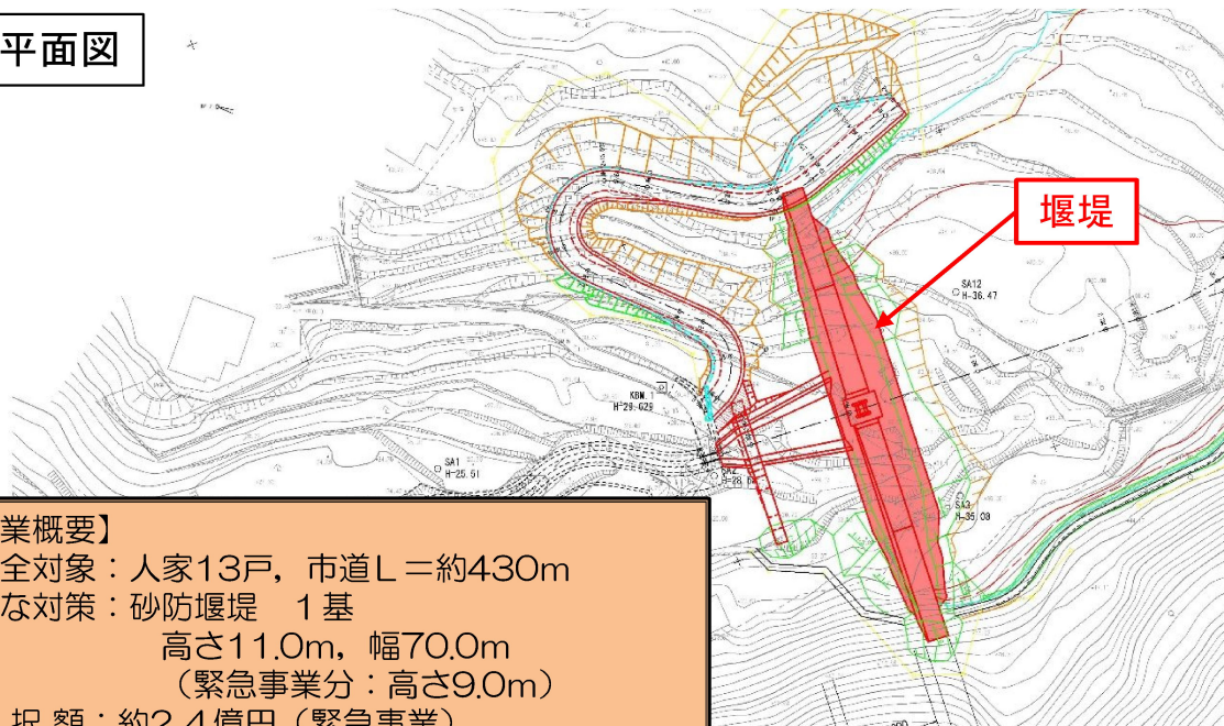
堰堤一般図
