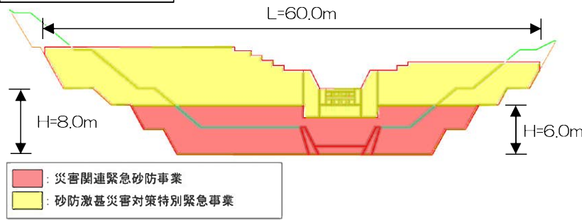
堰堤一般図
