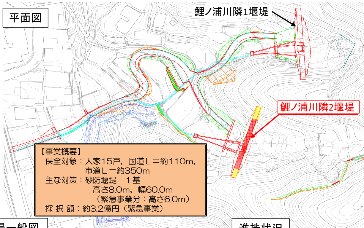
堰堤一般図
