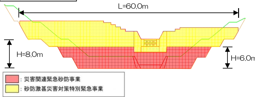
堰堤一般図
