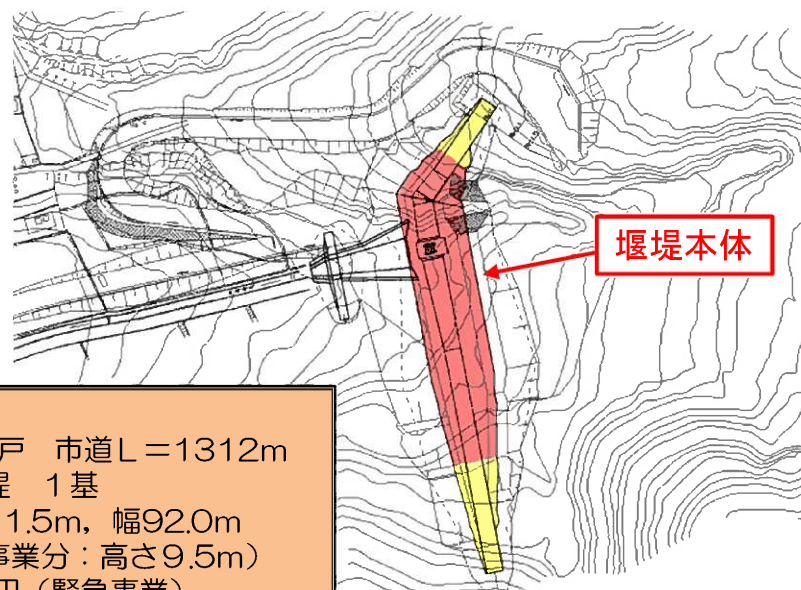
平面図
